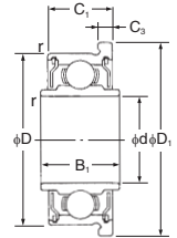
防尘盖型 ZZ · ZZS
