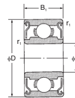
防尘盖型 ZZ·ZZ1
