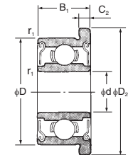
防尘盖型 ZZ · ZZ1
